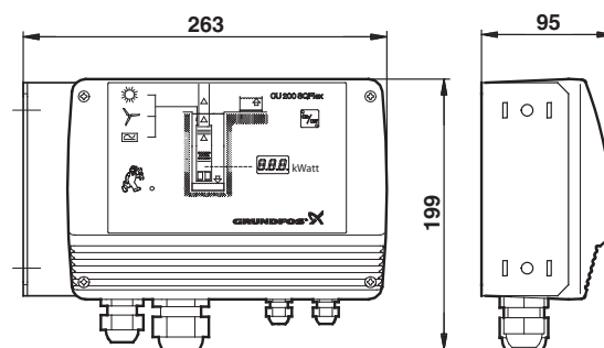
Fig. 19 Dimensions, CU 200
